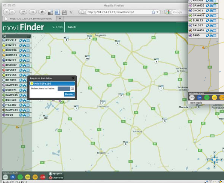
RECORRIDOS HISTÓRICOS
