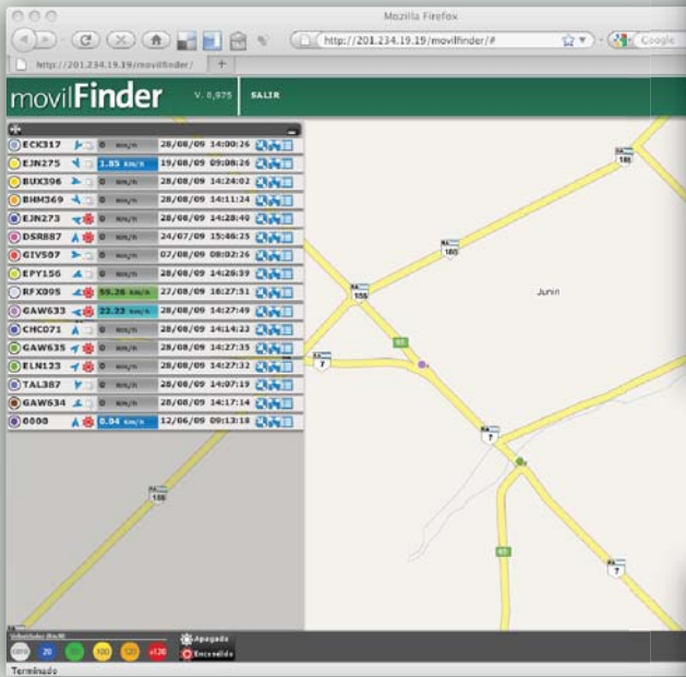
MÚLTIPLES MÓVILES
